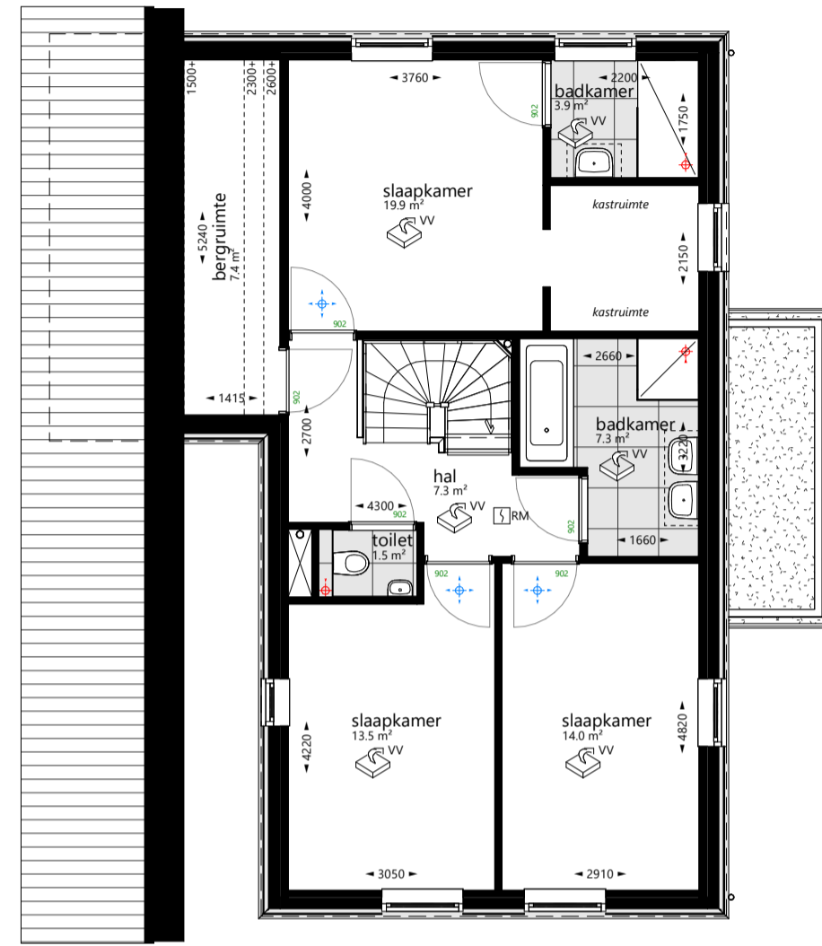
plattegrond 1e verdieping
