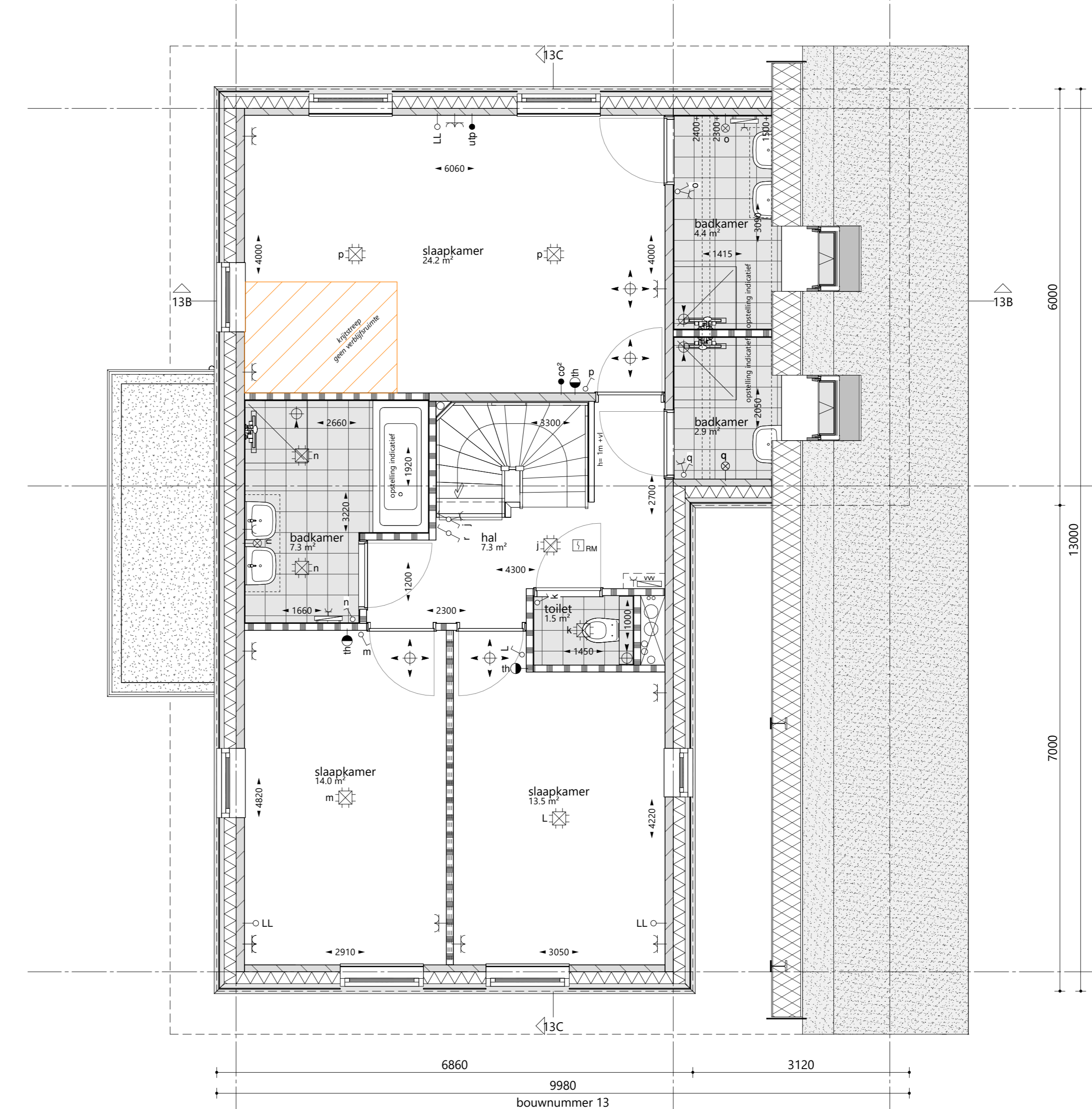
1e verdieping 1 : 50 optie: 2x dakraam zijgevel 0,94 x 1,40 m optie: uitwisseling (hoofd)badkamer + inloopkast optie: extra badkamer
