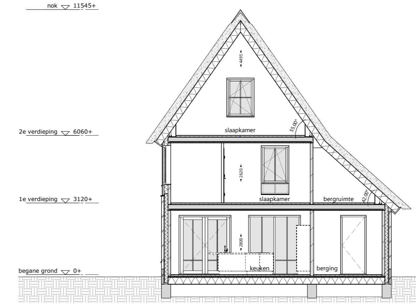
dwarsdoorsnede B 1 : 100
