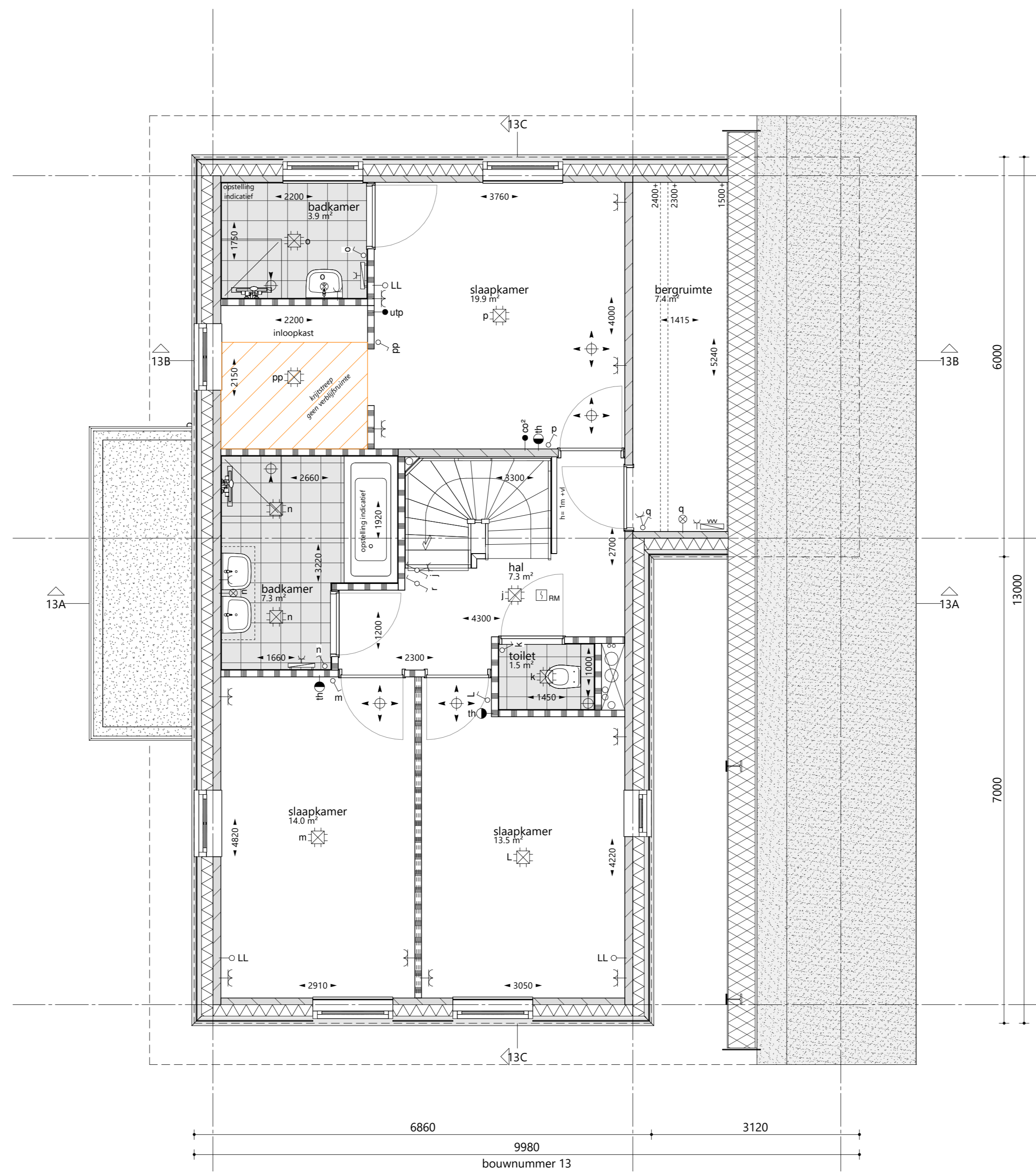
1e verdieping 1 : 50
