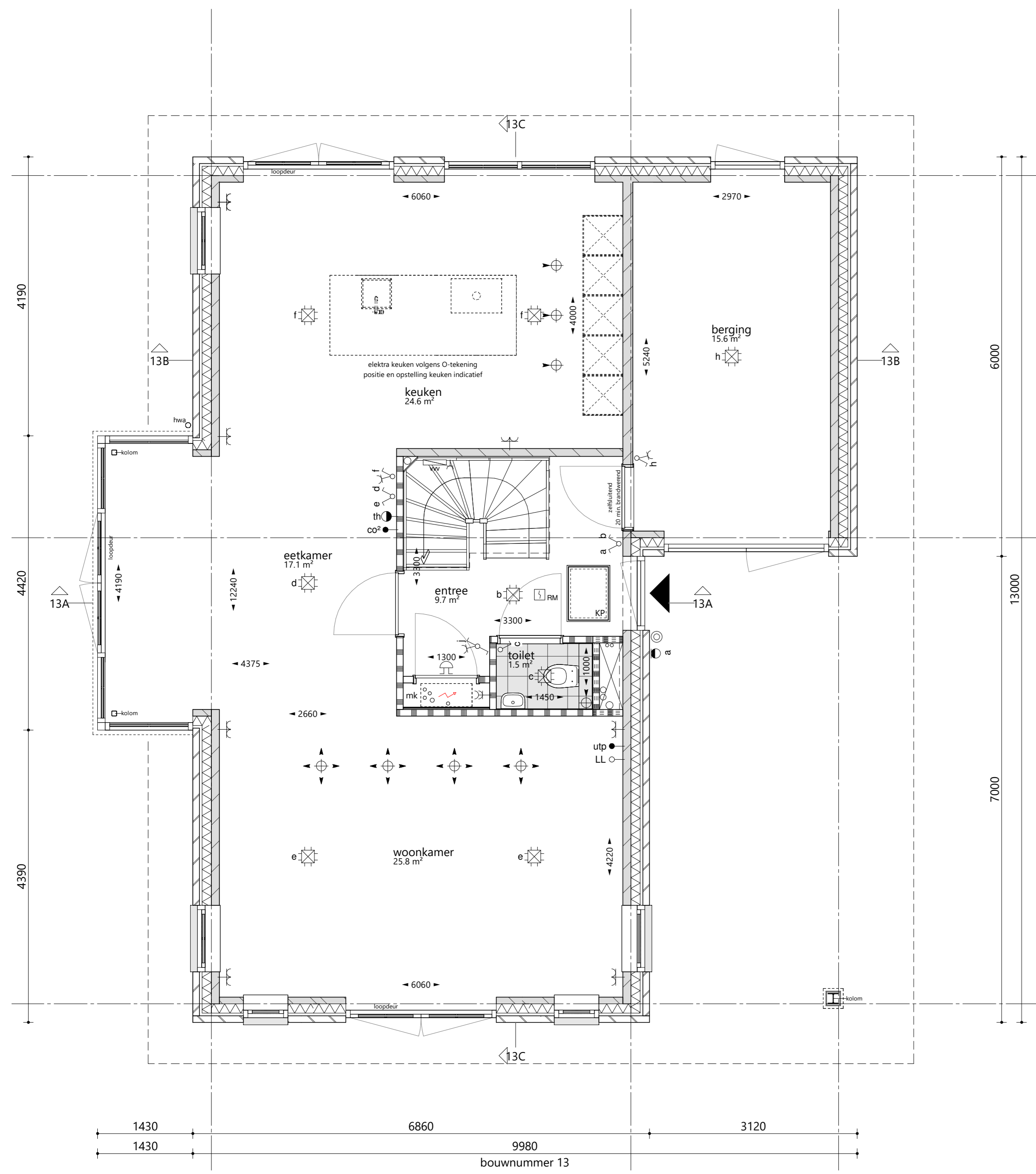
begane grond 1 : 50
