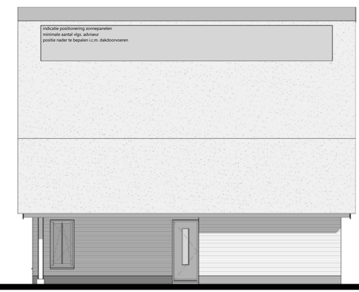
rechtergevel 1 : 100
