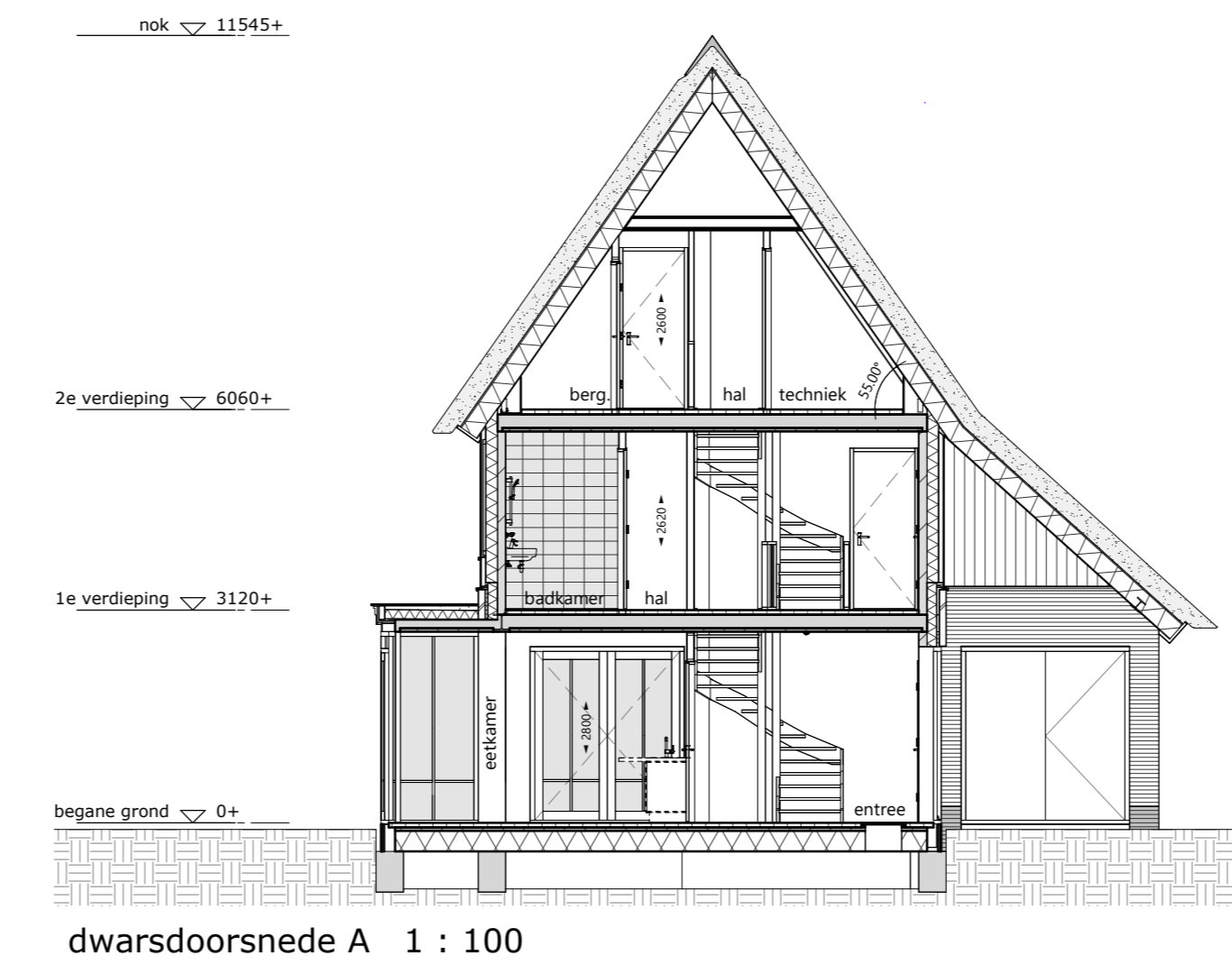
dwarsdoorsnede A 1 : 100
