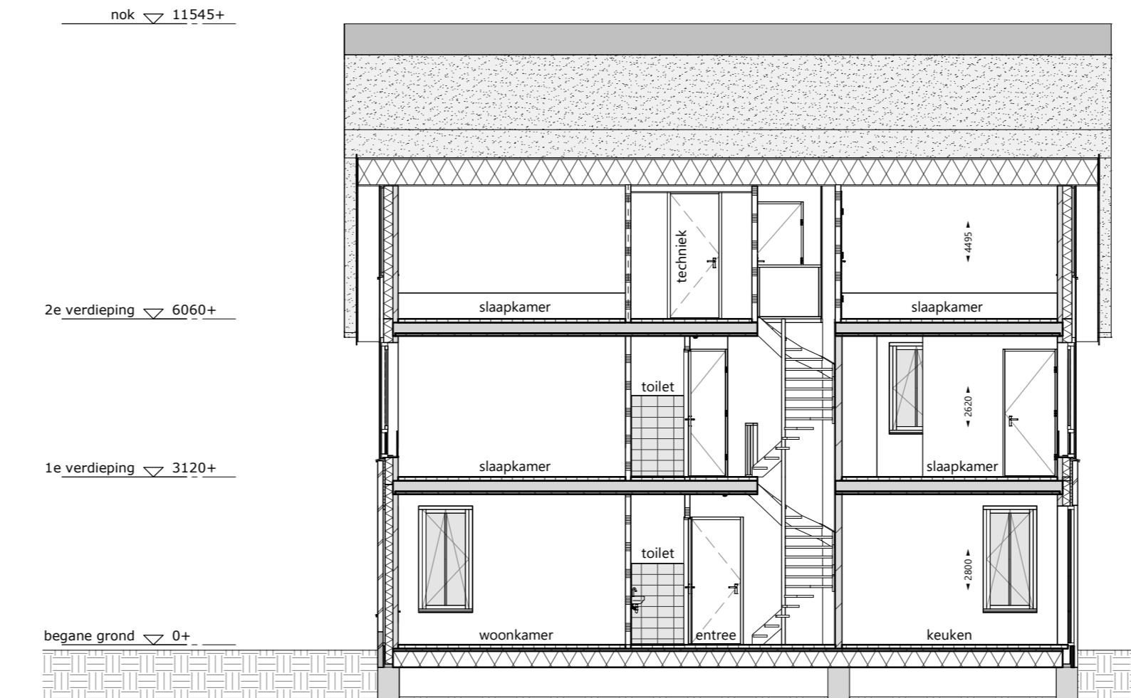
langsdoorsnede C 1 : 100
