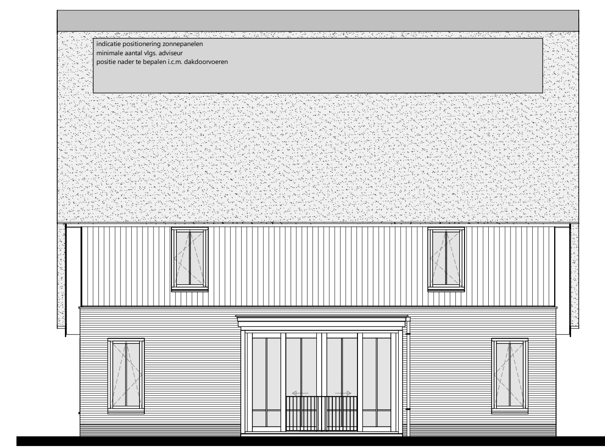
rechtgervel 1 : 100
