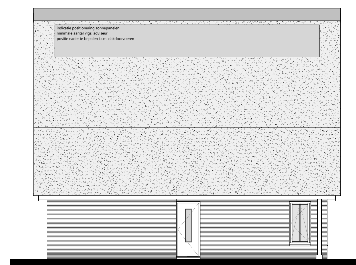
linkergevel 1 : 100
