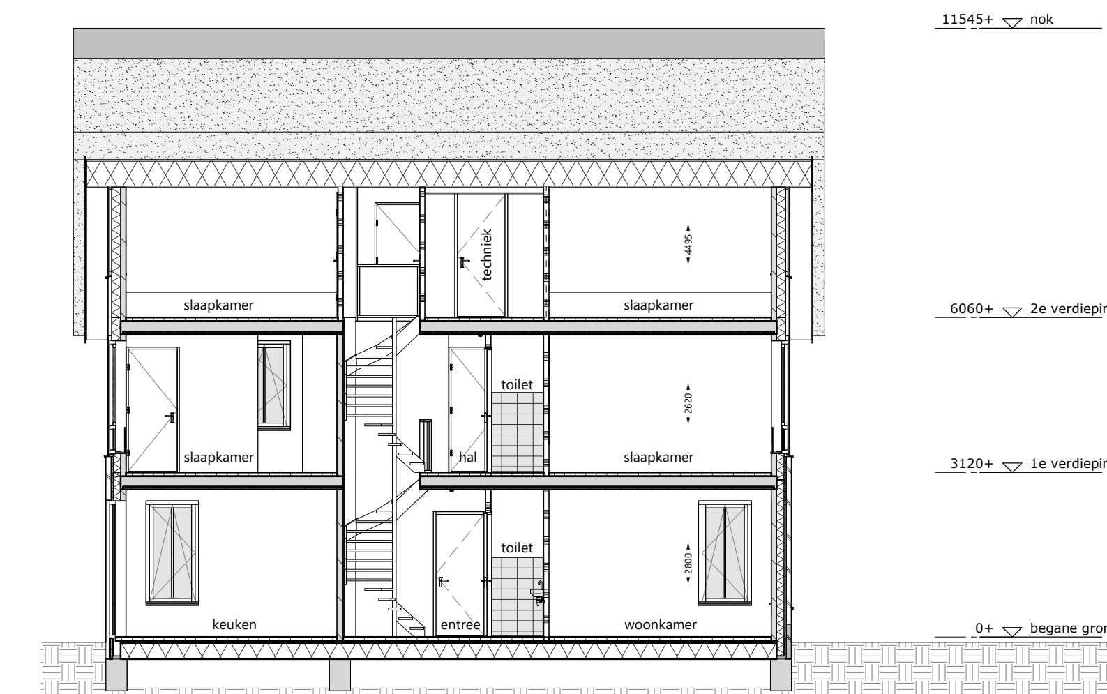
langsdoorsnede C 1 : 100
