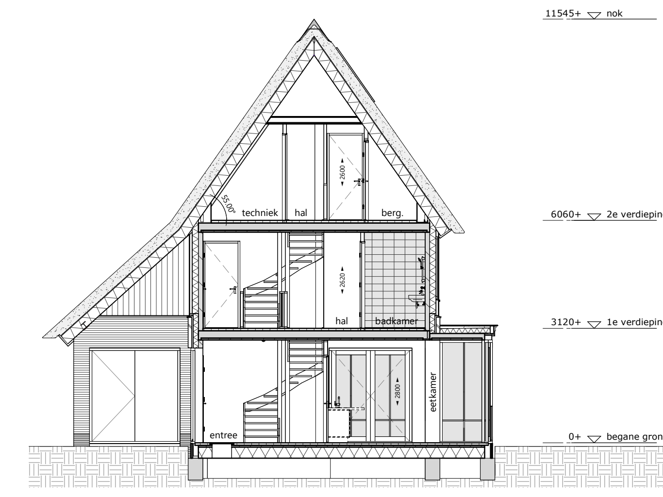
dwarsdoorsnede A 1 : 100
