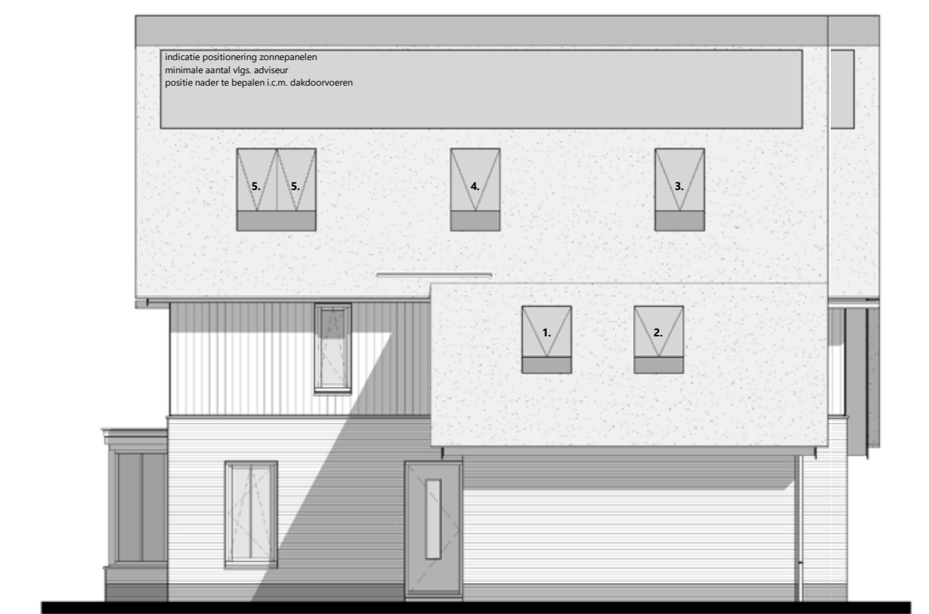
rechtergevel 1 : 100
