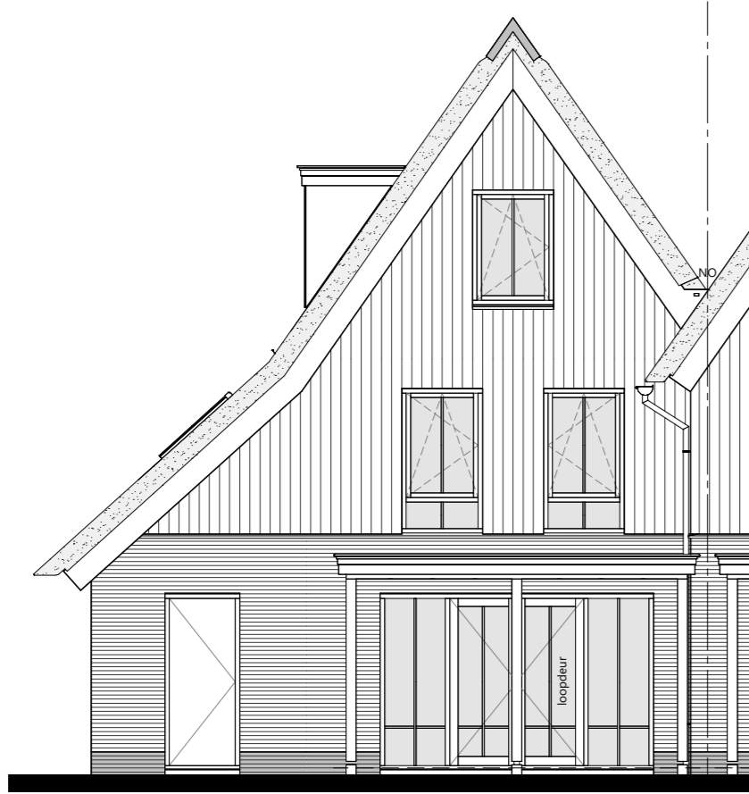
achtergevel 1 : 100 optie: veranda achtergevel 1,20 x 5,06 m optie: veranda achtergevel 2,40 x 5,06 m optie: dakkapel(len) zijgevel
