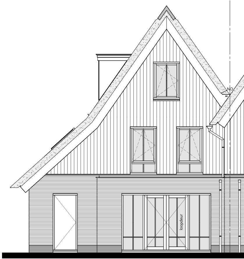
achtergevel 1 : 100 optie: aanbouw achtergevel 2,40 x 6,40 m optie: dakkapel(len) zijgevel
