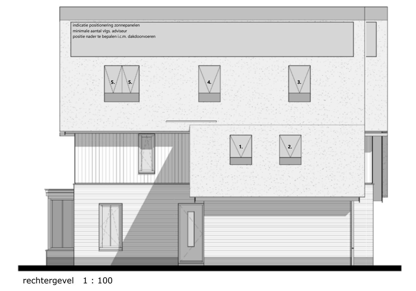
opties dakramen bouwnummers: 01, 02, 05, 06 1. enkel dakraam bergruimte 0,94 x 1,40 m 2. enkel dakraam bergruimte 0,94 x 1,40 m 3. enkel dakraam slaapkamer 0,94 x 1,40 m 4. enkel dakraam hal 0,94 x 1,40 m 5. dubbel dakraam slaapkamer 1,51 x 1,40 m (opties dakramen indicatief)
