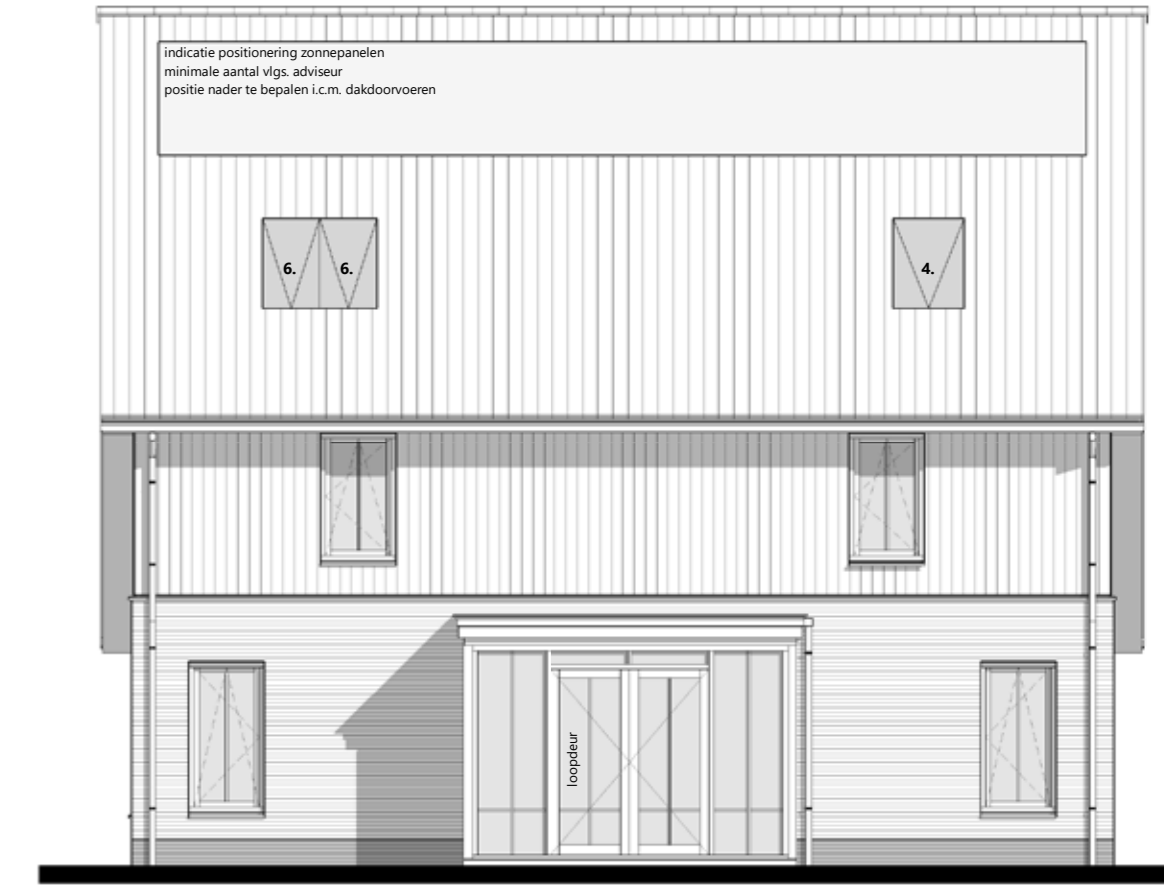
rechtgevel 1 : 100
